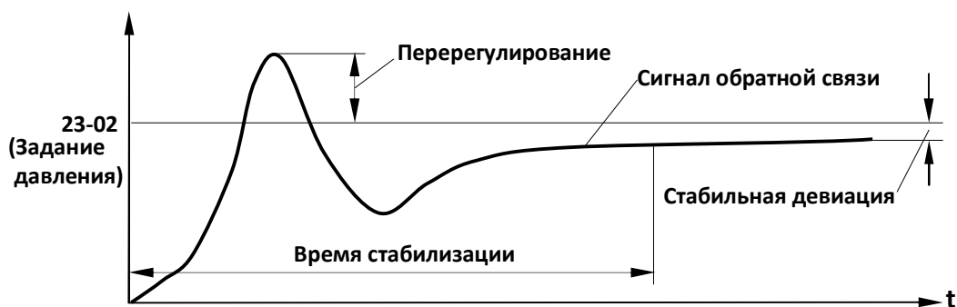
Диаграмма сигнала обратной связи
