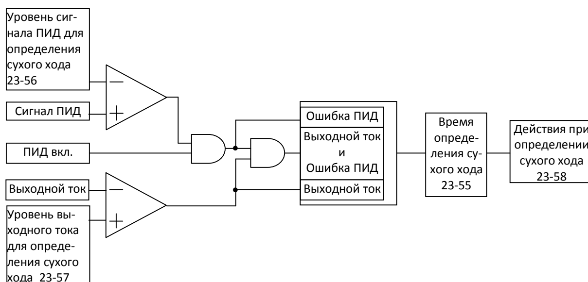
Блок-схема алгоритма реакции ПЧ на сухой ход.
