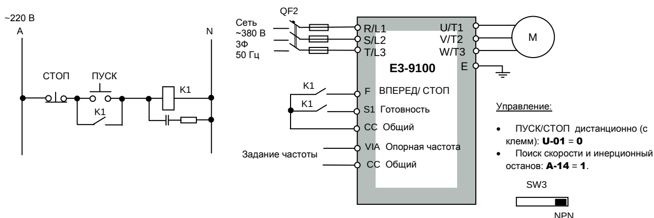
Схема управления воздухоудвкой пылеуловителя
