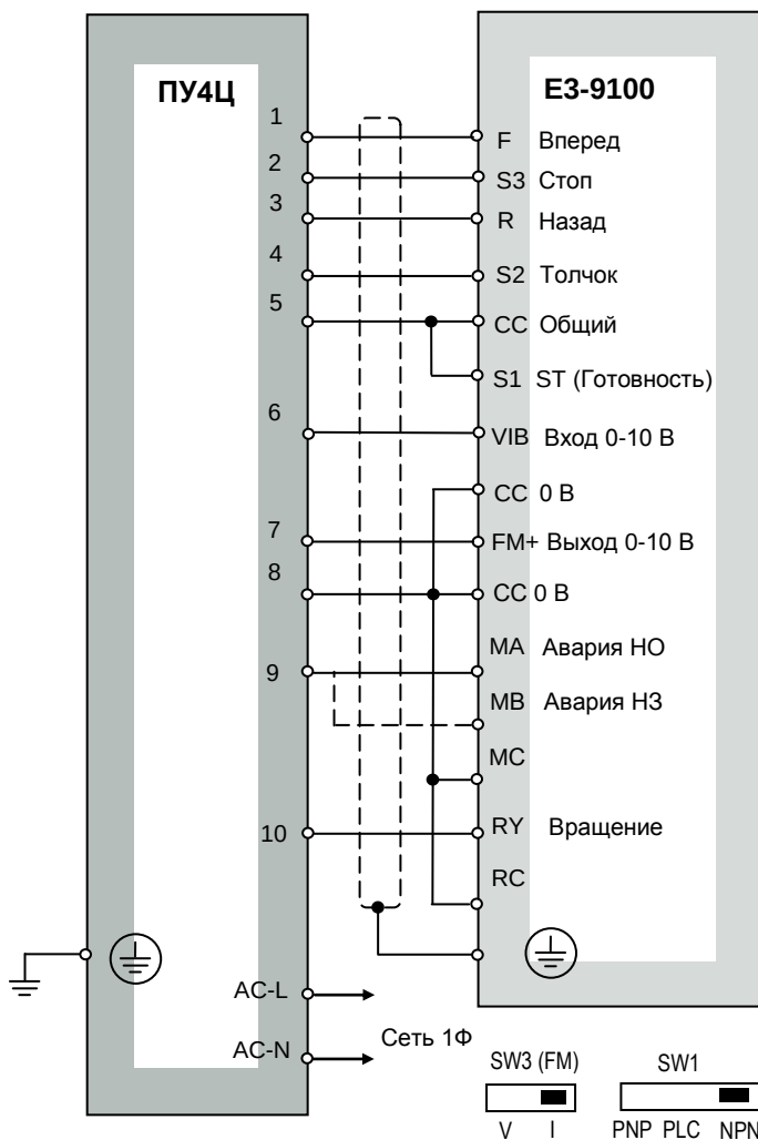
Подключение пульта ПУ4Ц к преобразователю ЕЗ-9100
