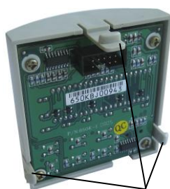
Фиксаторы пульта для крепления в монтажной рамке
