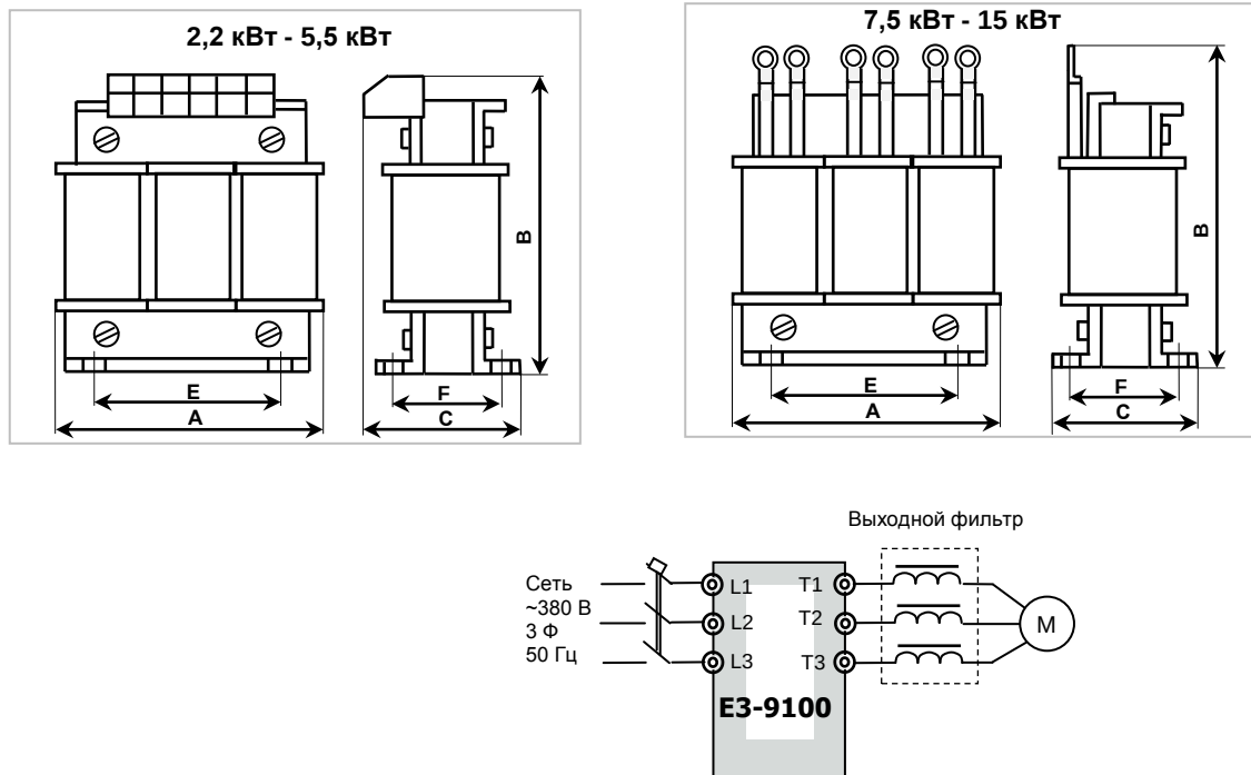
Схема включения выходного фильтра
