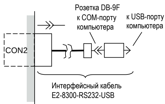
Подключение интерфейсного кабеля E2-8300-RS232-USB
